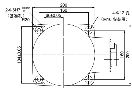
底座安装面 (从上面观察)
