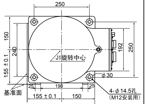
底座安装尺寸 (B-B视图)
