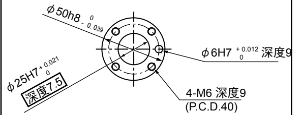
工具安装面详图 (A视图)
