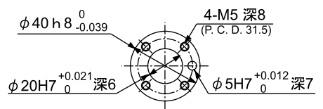
ツール取付面詳細 (矢視A)
