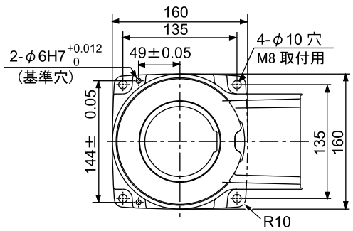
ベース取付寸法 (上面より)
